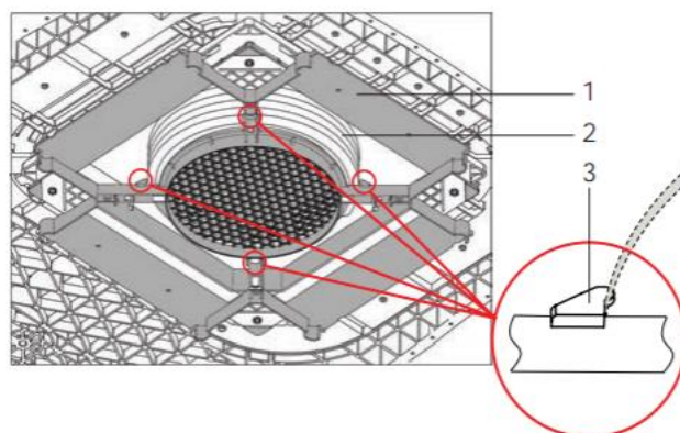
Рис.16. Закрепление воздуховода
