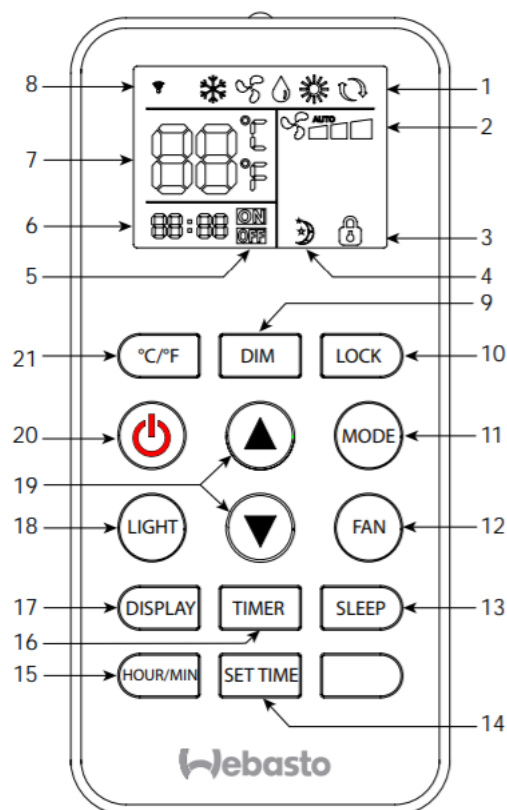
Рис.23. Пульт дистанционного управления
