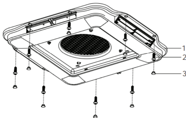
Рис.21. Дополнительная фиксация воздухораспределительного модуля
