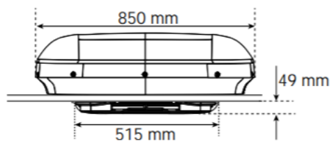
Рис.6. Вид спереди
