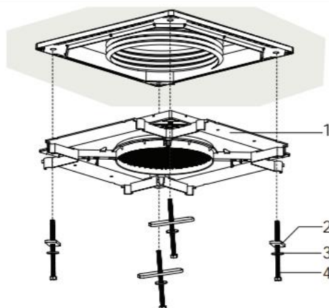
Рис.15. Установка крепежных болтов
