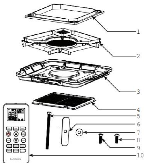
Рис.2. Салонный блок
