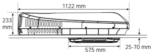
Рис.5. Вид сбоку
