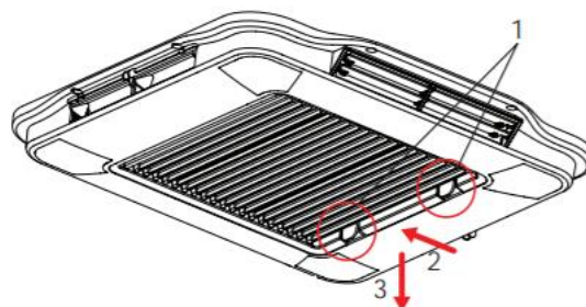
Рис.17. Воздухораспределительный модуль
