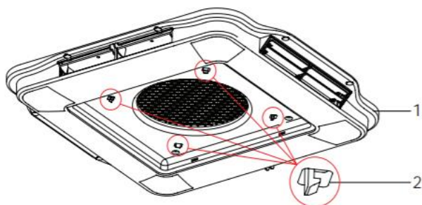
Рис.19. Установка воздухораспределительного модуля
