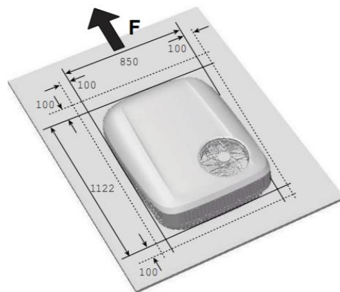
Рис.3. Монтажное положение накрывного блока
