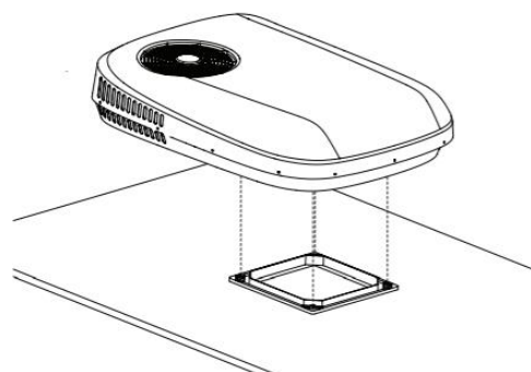
Рис.13. Установка накрышного блока
