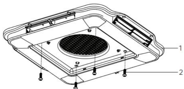
Рис.20. Фиксация воздухораспределительного модуля
