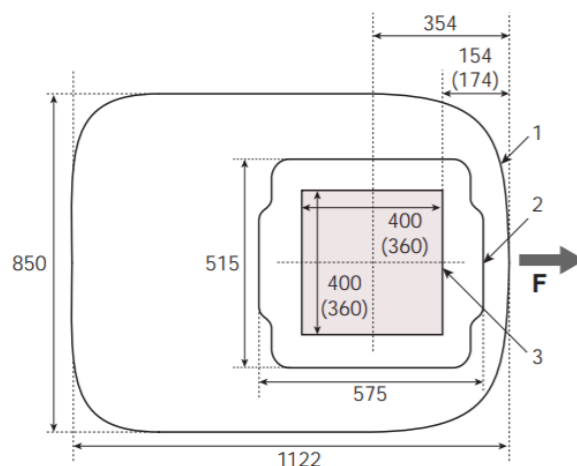
Рис.4. Разметка на крыше
