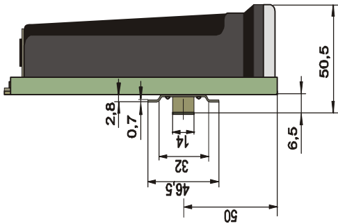
Рисунок 6 - Блок управления
