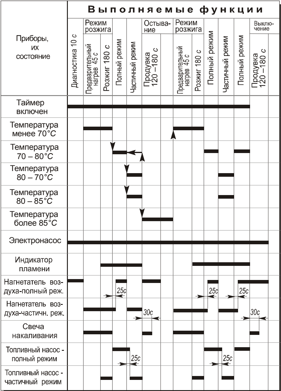
Рисунок 2 - Диаграмма работы подогревателя.
